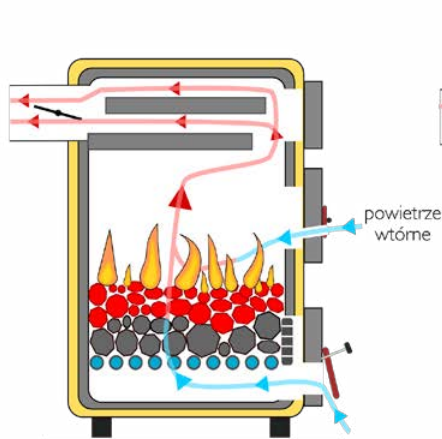
Kocioł z poziomym wymiennikiem
