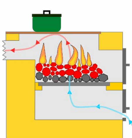
Piec kuchenny
