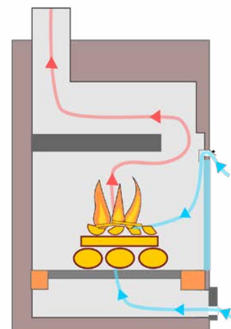
Kominiek / piec na drewno
