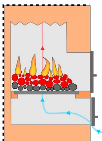
Piec kaflowy
