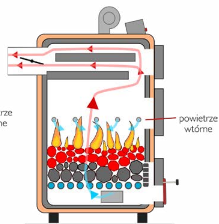
Kocioł z nadmuchem
