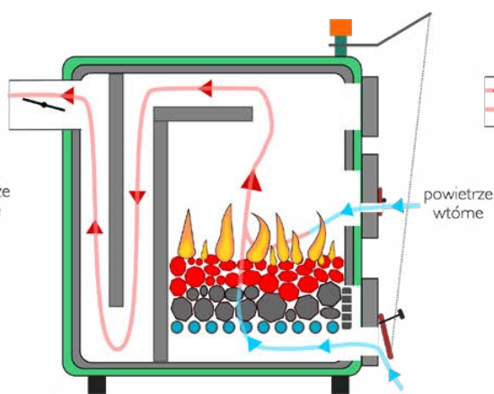
Kocioł z pionowym wymiennikiem
